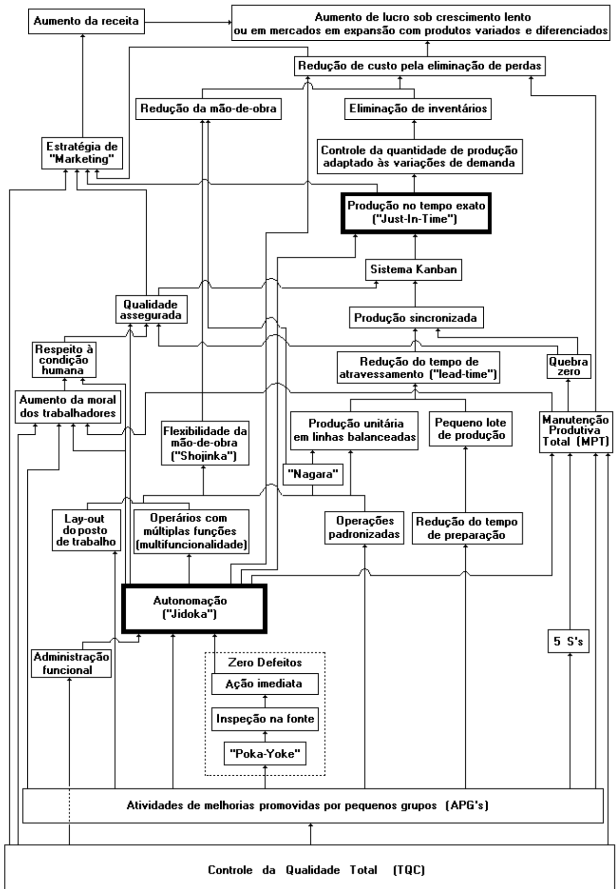
FIGURA 3 - ESTRUTURA DO SISTEMA TOYOTA DE PRODUÇÃO PROPOSTA PELA PESQUISA
